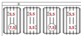
VÝKON HOŘÁKŮ
